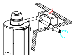
Scarico Sdoppiato
